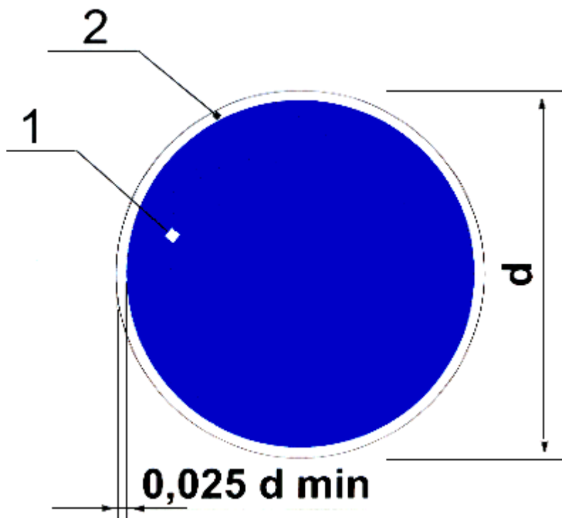
Рисунок 3 - Основа цветографического изображения и соотношение размеров предписывающих знаков безопасности
