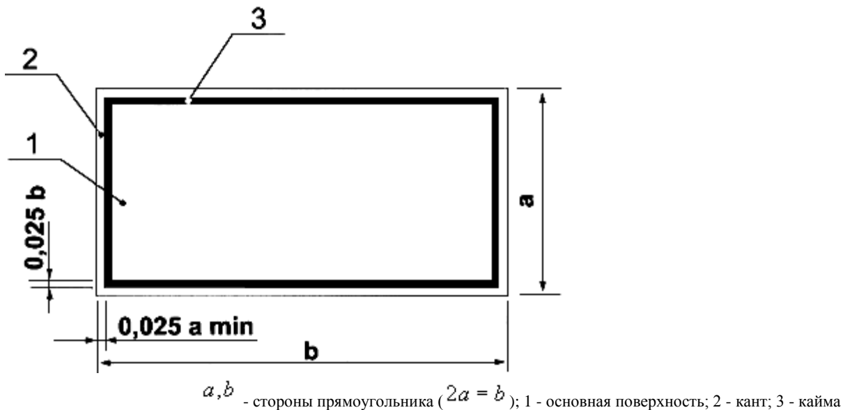
Рисунок 7 - Основа цветографического изображения и соотношение размеров дополнительных знаков безопасности
