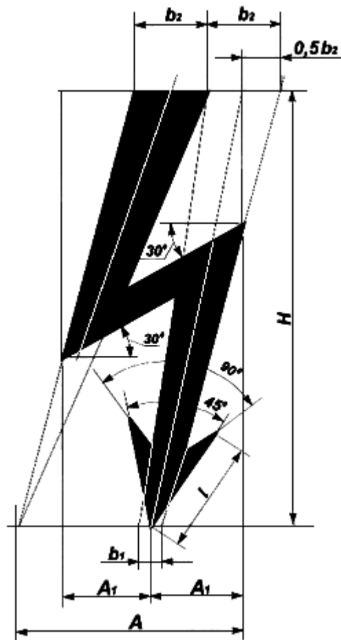
Рисунок Л.1 - Графический символ электрического напряжения
